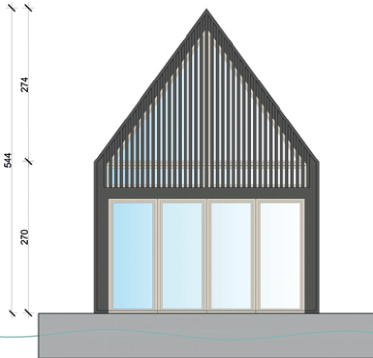
TOP ELEVATION
