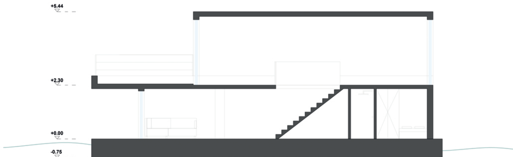
SECTION A-A
