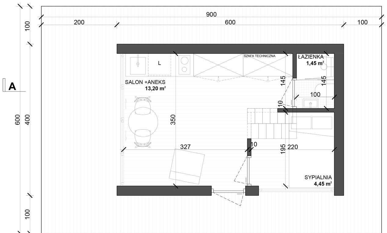
RZUT PARTERU
